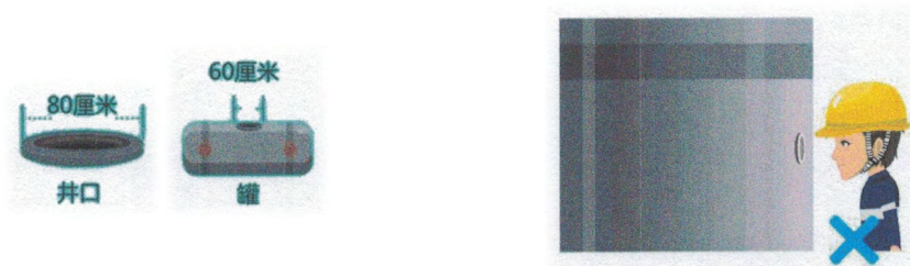
(a) 直径 80 cm 的井口或直径 60 cm 的人孔 (b) 设有观察孔的储罐
