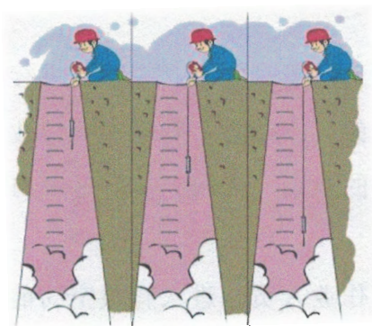
图 4-5 垂直方向气体检测
